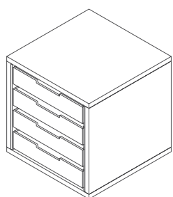
Construction MDF de 18 mm. 4 plateaux acryliques. 369x369x400 mm / 48 Ø STK.WBT4 340,00 €
